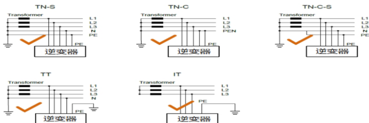
图 2.2 光伏并网逆变器支持的电网形式
