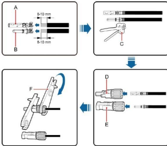
图 5.2 MC4 直流连接器与光伏组串的连接
