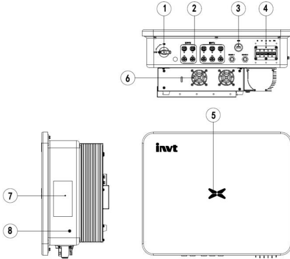
图 2.3 三相光伏逆变器外观图
