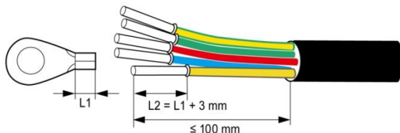
图 5.5 压接电缆端子
