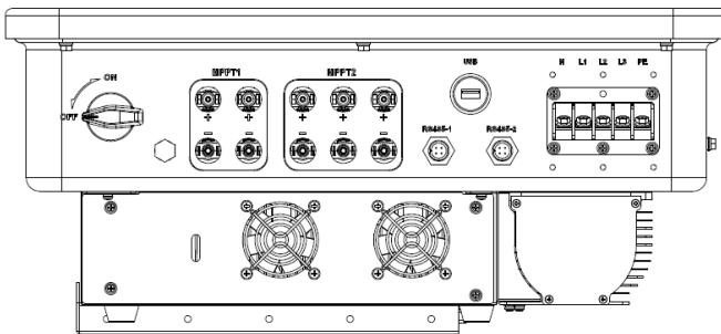
YG15-25KTR 底部示意图
