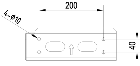
图 4.6 安装挂板尺寸图
