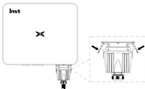
图 5.7 AC 防水罩卡扣固定
